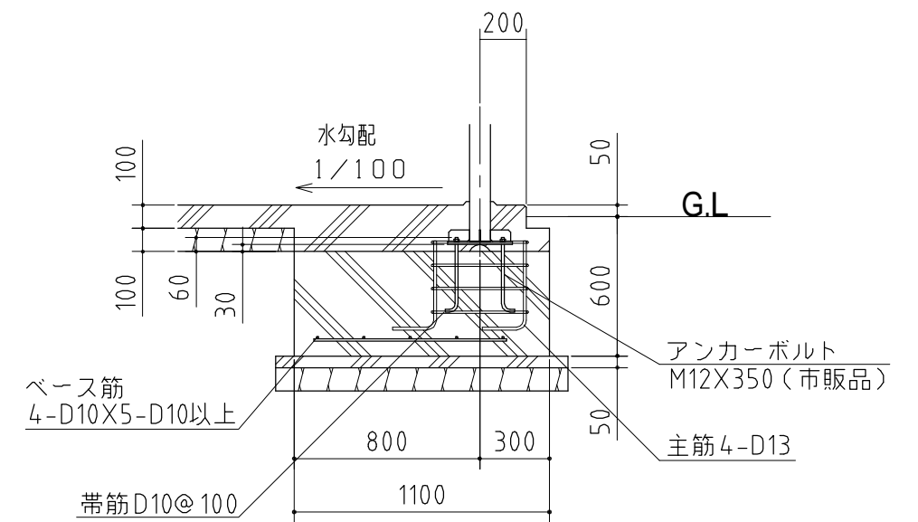
A-A' 断面
